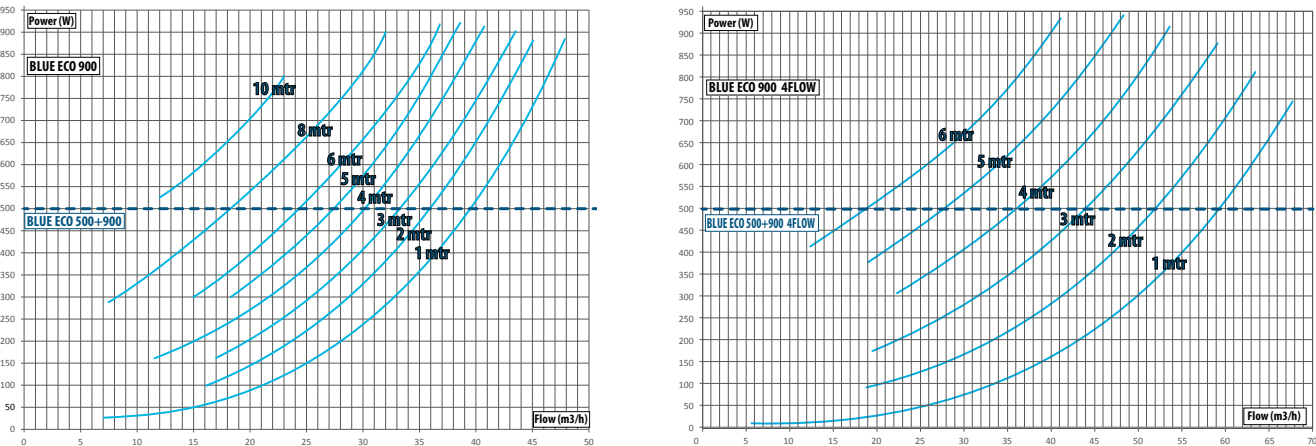
In deze grafiek is de pompcurve te zien van de Blue Eco 500 en 900 (met en zonder 4Flow pompkop) bij verschillende opvoerhoogtes. De scheidslijn bij 500 watt geeft aan waar de capaciteit van de Blue Eco 500 watt ophoudt, boven deze lijn geldt alleen voor de Blue Eco 900.
